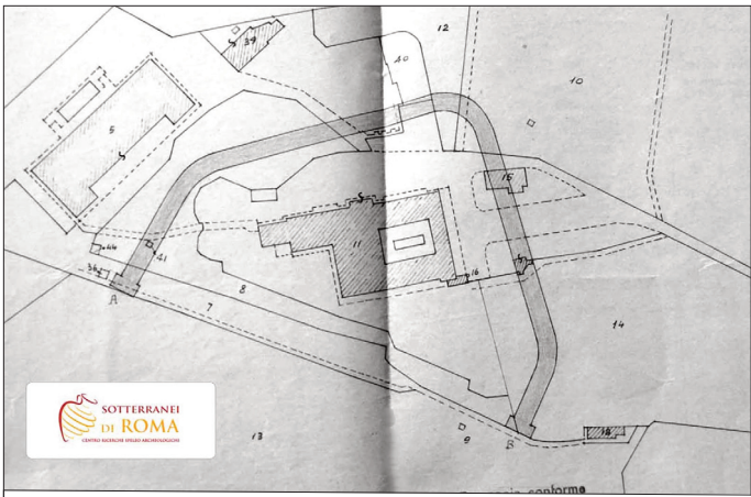
FOTO 3 Planimetria del rifugio. (Foto concessa Sotteranei di Roma)
